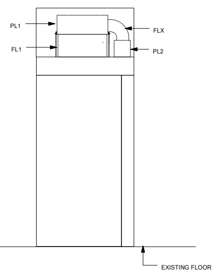
ELEVATION "C"
