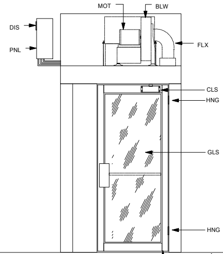
ELEVATION "C"
